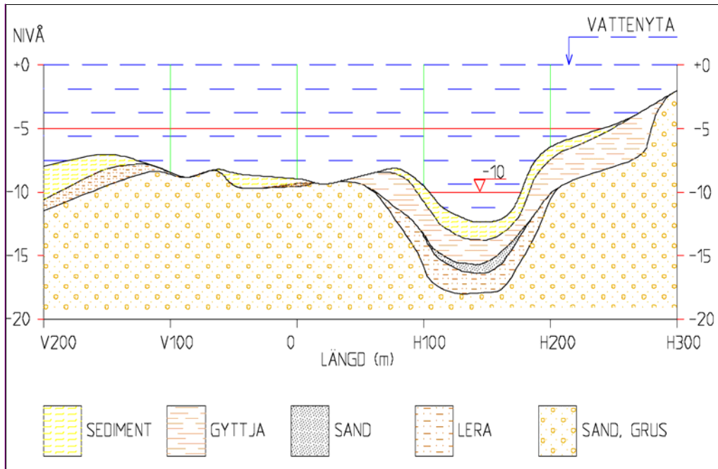
Figur 3. Schematisk bild av jordlagerföljd och en tänkbar fördelning av sediment i tvärsnittet.
